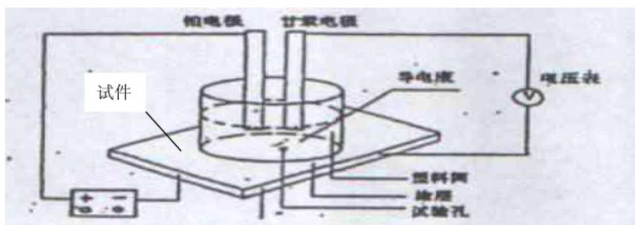
图 B.0.3 防腐层阴极剥离试验示意图
